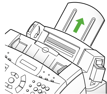
Afdrukpapiersteun uitschuiven
